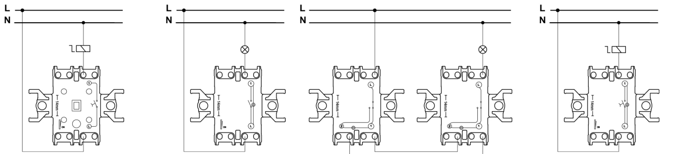
Кнопочный выключатель
