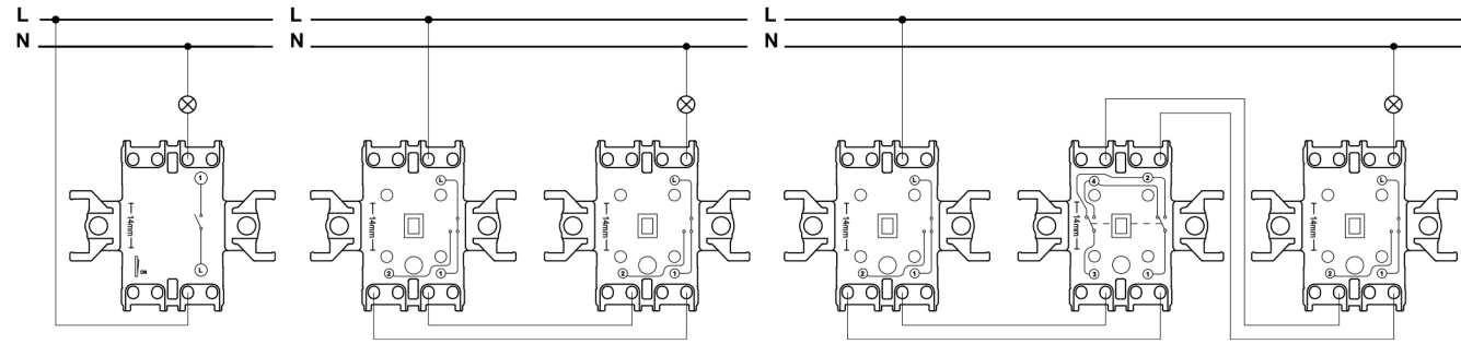
Одноклавишный выключатель
