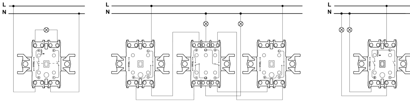
Двухполюсный выключатель
