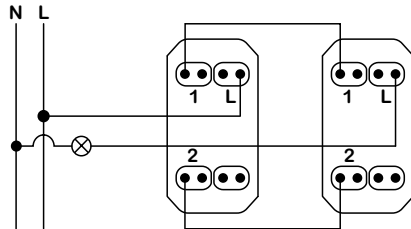
1 модуль – 2 переключателя
