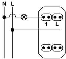
1 модуль – выключатель
